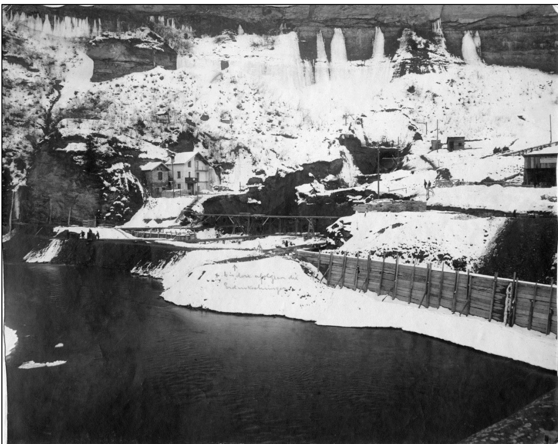
Barrage de la Maigrauge : construction de l'usine de l'Oelberg ; Photographe inconnu ; 1909. SALV : © Bibliothèque cantonale et universitaire Fribourg. Fonds Salvisberg (Usine de l'Oelberg).
