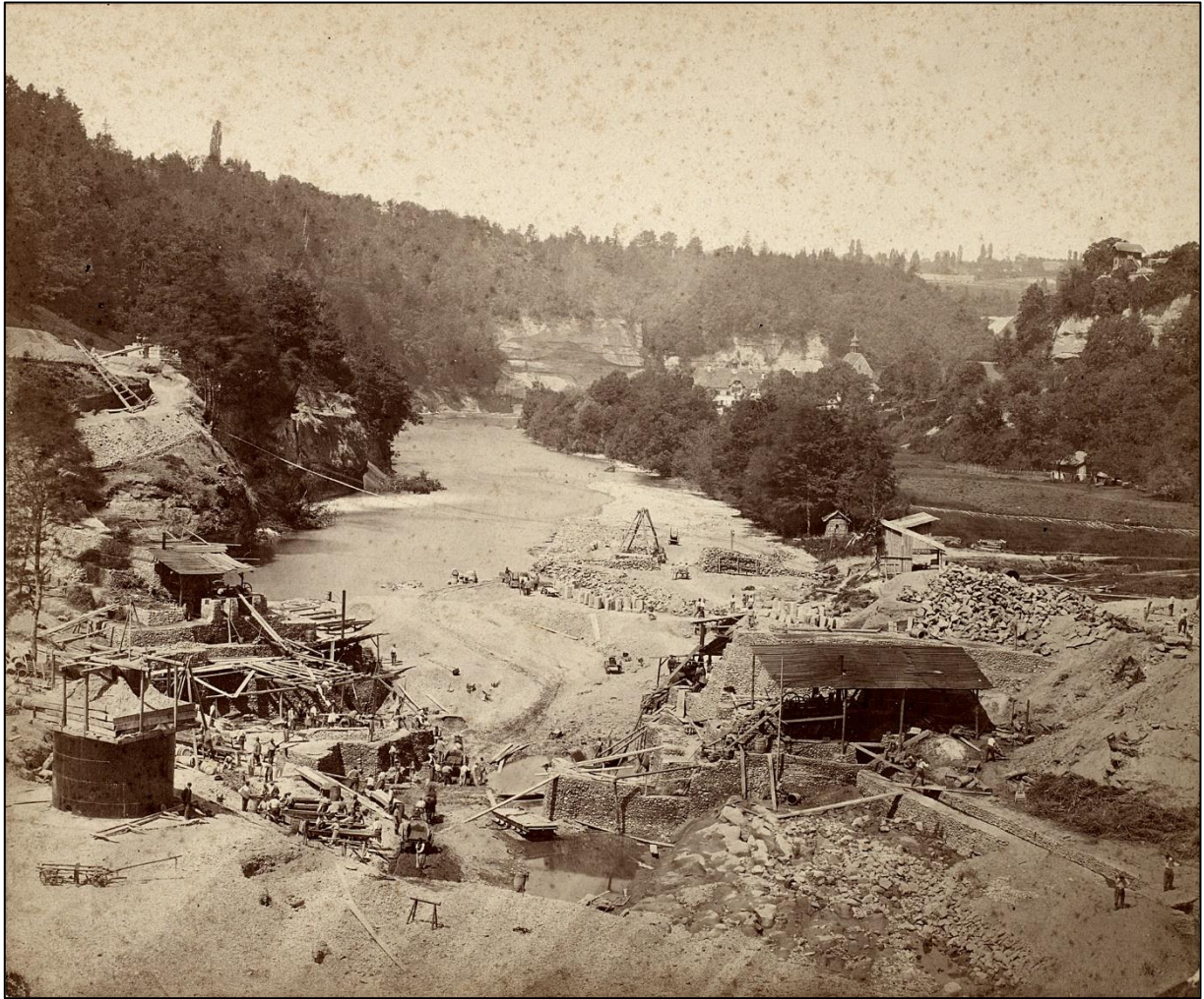
Construction du barrage de la Maigrage ; Photographie inconnu ; entre 1870 et 1872. PHCA : © Bibliothèque cantonale et universitaire Fribourg. Collection de photos sur carton.
