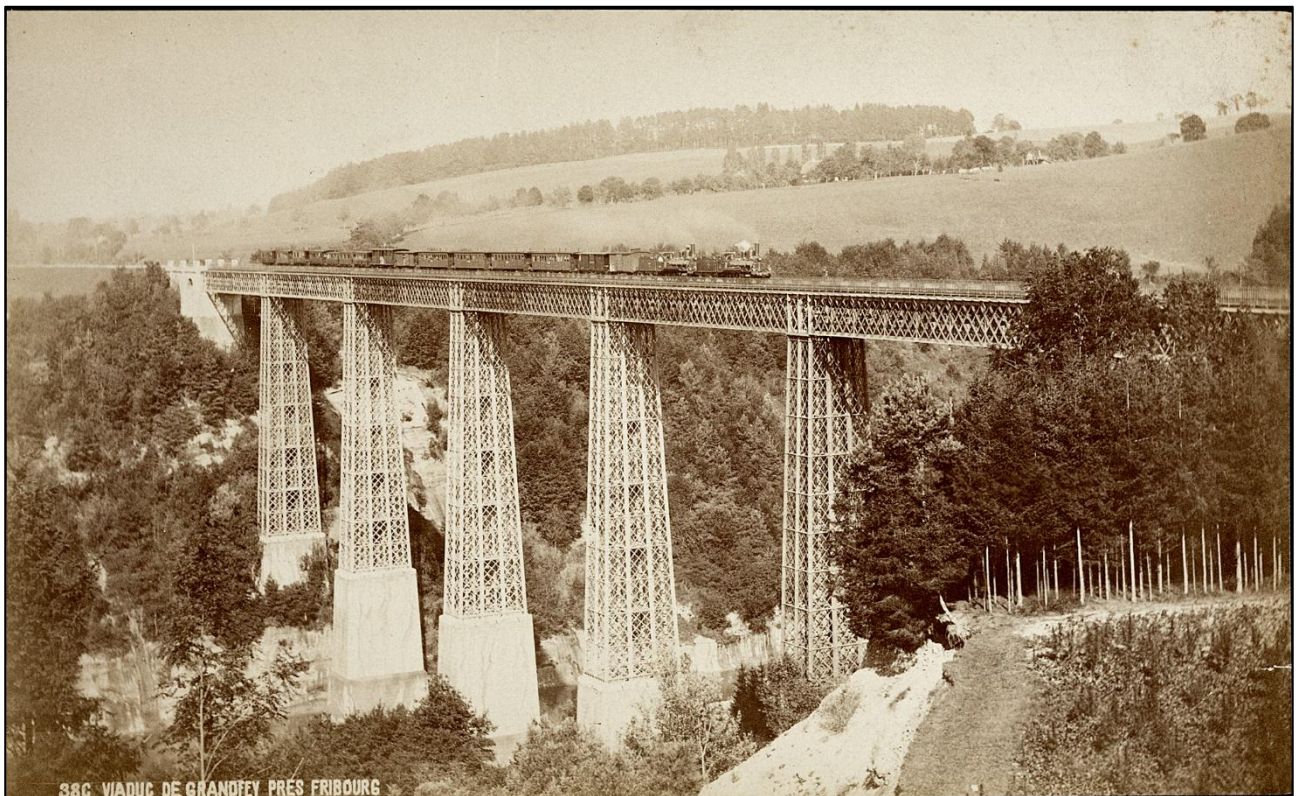
Pont ou viaduc de Grandfey et train à vapeur ; Jullien, John ; ca. 1880. PHCA : © Bibliothèque cantonale et universitaire Fribourg. Collection de photos sur carton.
